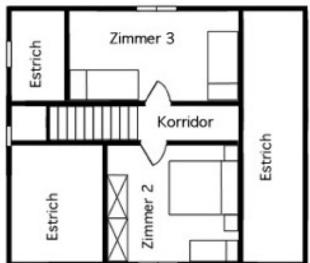
obere Etage
